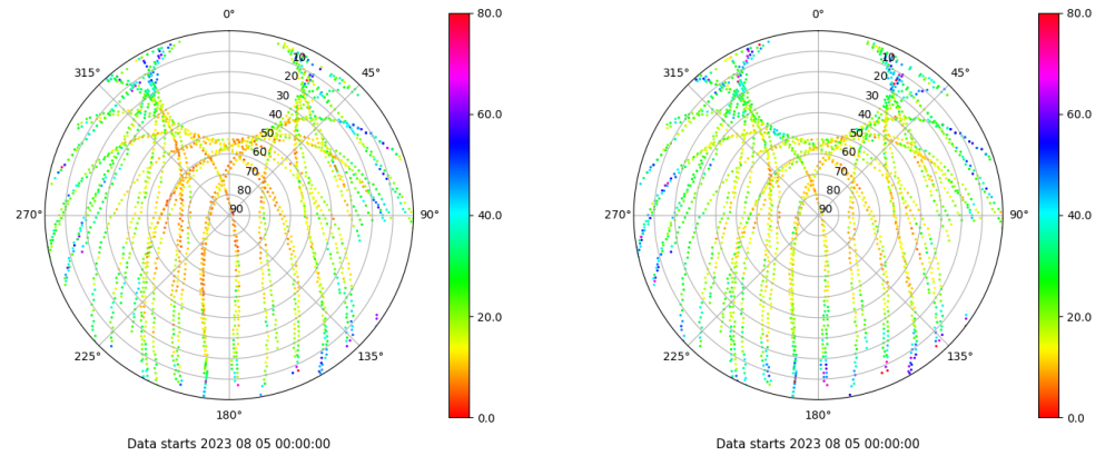
Skyplot for station CAAL. Parameter M1C Data file CAAL00ESP_R_2023217.xtr Skyplot for station CAAL. Parameter M2P Data file CAAL00ESP_R_2023217.xtr
