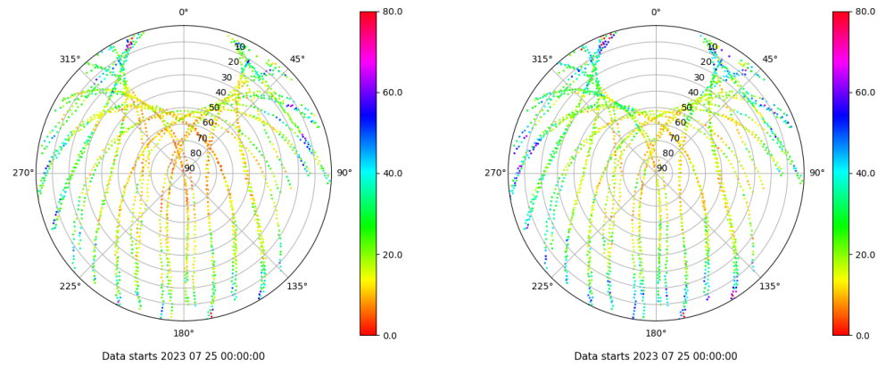
Skyplot for station CAAL. Parameter M1C Data file CAAL00ESP_R_2023206.xtr Skyplot for station CAAL. Parameter M2P Data file CAAL00ESP_R_2023206.xtr
