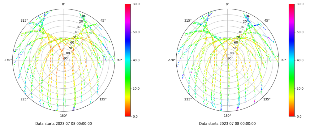
Skyplot for station CAAL. Parameter M1C Data file CAAL00ESP_R_2023189.xtr Skyplot for station CAAL. Parameter M2P Data file CAAL00ESP_R_2023189.xtr
