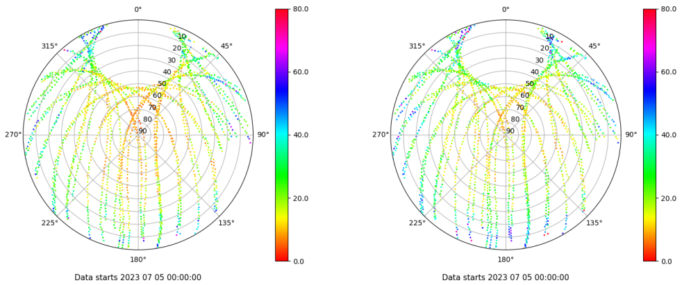
Skyplot for station CAAL. Parameter M1C Data file CAAL00ESP_R_2023186.xtr Skyplot for station CAAL. Parameter M2P Data file CAAL00ESP_R_2023186.xtr
