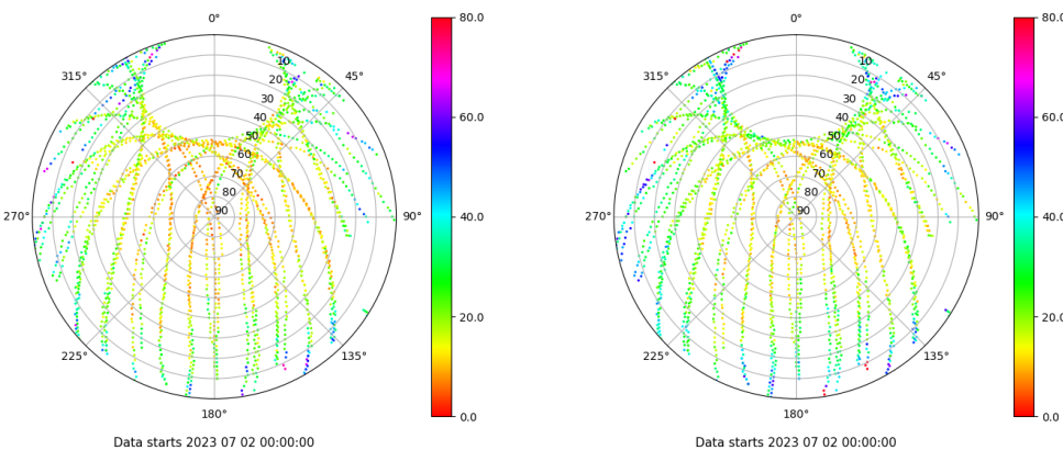
Skyplot for station CAAL. Parameter M1C Data file CAAL00ESP_R_2023183.xtr Skyplot for station CAAL. Parameter M2P Data file CAAL00ESP_R_2023183.xtr
