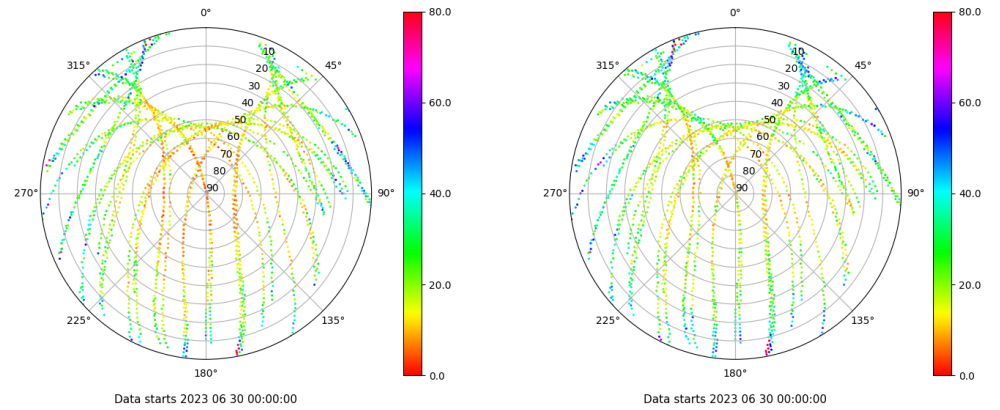
Skyplot for station CAAL. Parameter M1C Data file CAAL00ESP_R_2023181.xtr Skyplot for station CAAL. Parameter M2P Data file CAAL00ESP_R_2023181.xtr
