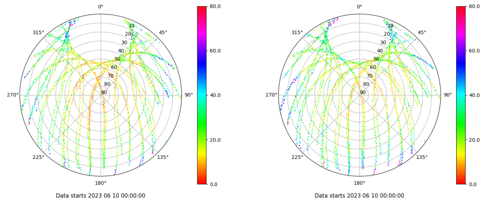
Skyplot for station CAAL. Parameter M1C Data file CAAL00ESP_R_2023161.xtr Skyplot for station CAAL. Parameter M2P Data file CAAL00ESP_R_2023161.xtr
