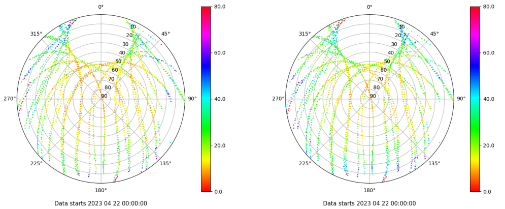
Skyplot for station CAAL. Parameter M1C Data file CAAL00ESP_R_2023112.xtr Skyplot for station CAAL. Parameter M2P Data file CAAL00ESP_R_2023112.xtr
