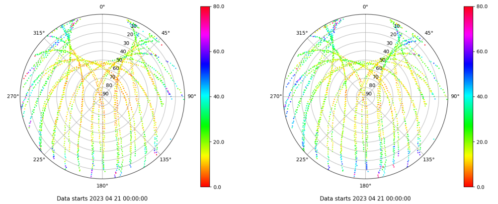
Skyplot for station CAAL. Parameter M1C Data file CAAL00ESP_R_2023111.xtr Skyplot for station CAAL. Parameter M2P Data file CAAL00ESP_R_2023111.xtr
