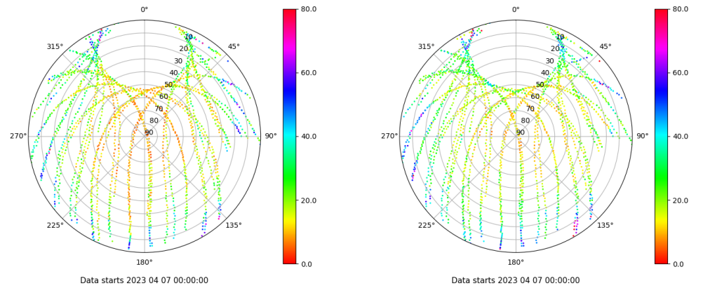
Skyplot for station CAAL. Parameter M1C Data file CAAL00ESP_R_2023097.xtr Skyplot for station CAAL. Parameter M2P Data file CAAL00ESP_R_2023097.xtr
