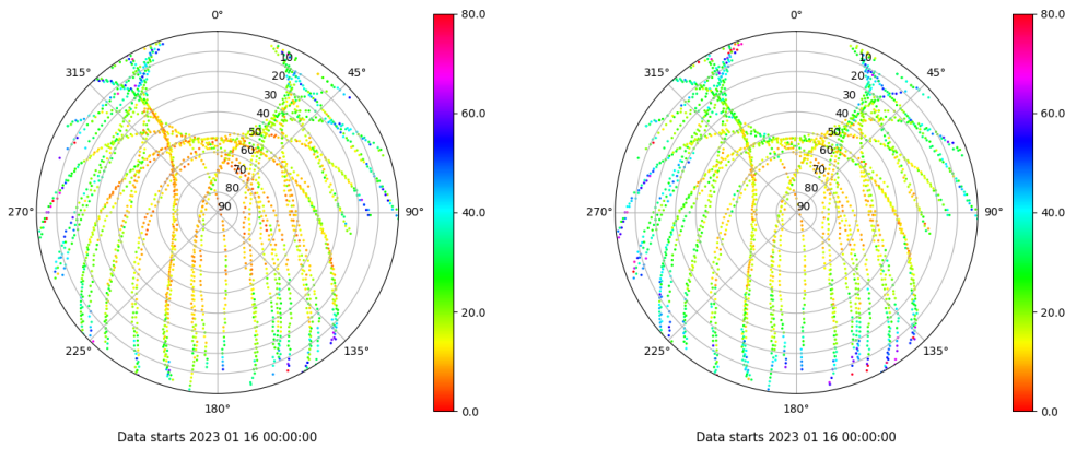
Skyplot for station CAAL. Parameter M1C Data file CAAL00ESP_R_2023016.xtr Skyplot for station CAAL. Parameter M2P Data file CAAL00ESP_R_2023016.xtr
