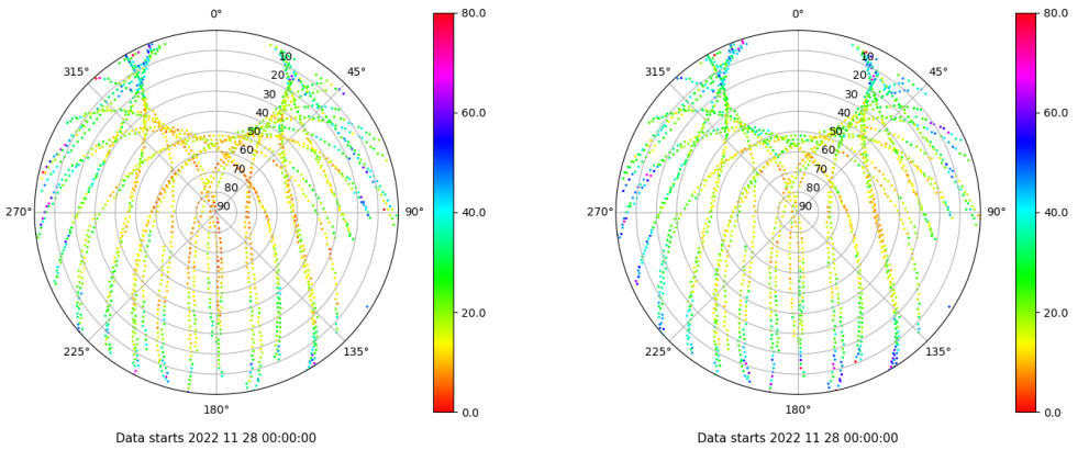
Skyplot for station CAAL. Parameter M1C Data file CAAL00ESP_R_2022332.xtr Skyplot for station CAAL. Parameter M2P Data file CAAL00ESP_R_2022332.xtr
