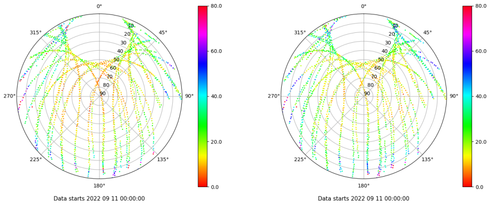
Skyplot for station CAAL. Parameter M1C Data file CAAL00ESP_R_2022254.xtr Skyplot for station CAAL. Parameter M2P Data file CAAL00ESP_R_2022254.xtr
