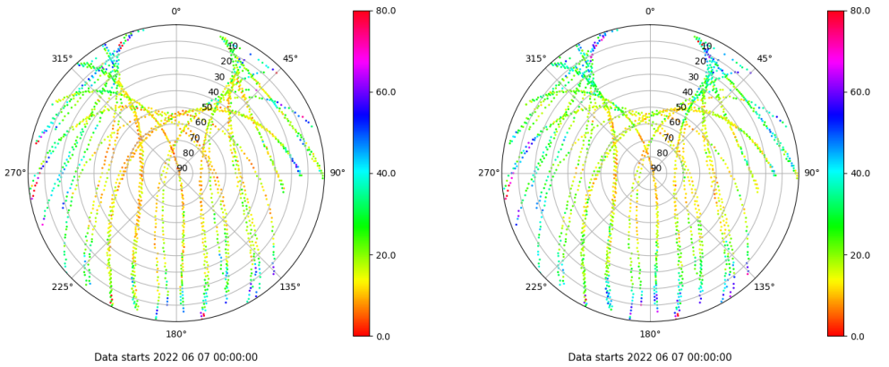
Skyplot for station CAAL. Parameter M1C Data file CAAL00ESP_R_2022158.xtr Skyplot for station CAAL. Parameter M2P Data file CAAL00ESP_R_2022158.xtr
