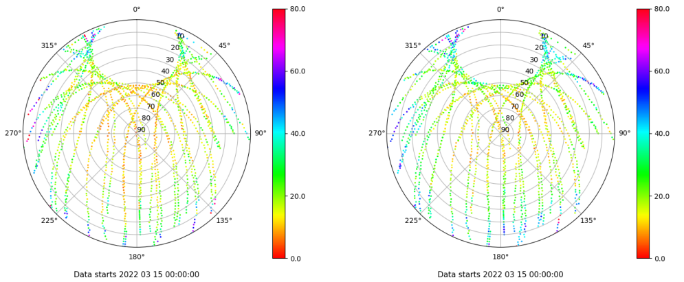
Skyplot for station CAAL. Parameter M1C Data file CAAL00ESP_R_2022074.xtr Skyplot for station CAAL. Parameter M2P Data file CAAL00ESP_R_2022074.xtr
