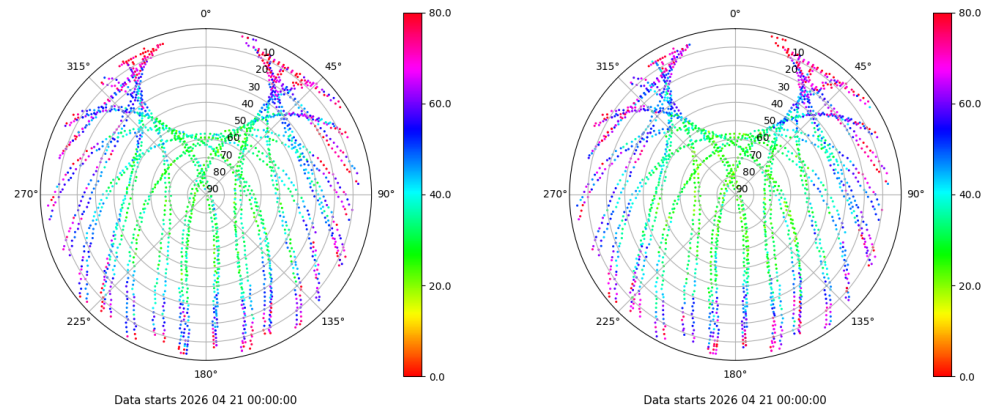
Skyplot for station BUIT. Parameter M1C Data file BUIT00ESP_R_2026111.xtr Skyplot for station BUIT. Parameter M2C Data file BUIT00ESP_R_2026111.xtr
