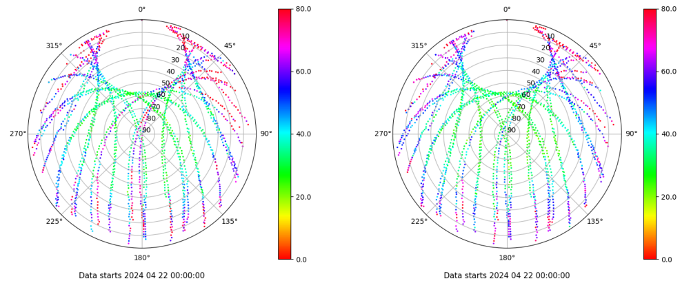
Skyplot for station BUIT. Parameter M1C Data file BUIT00ESP_R_2024113.xtr Skyplot for station BUIT. Parameter M2C Data file BUIT00ESP_R_2024113.xtr
