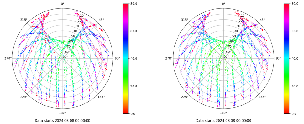
Skyplot for station BUIT. Parameter M1C Data file BUIT00ESP_R_2024068.xtr Skyplot for station BUIT. Parameter M2C Data file BUIT00ESP_R_2024068.xtr
