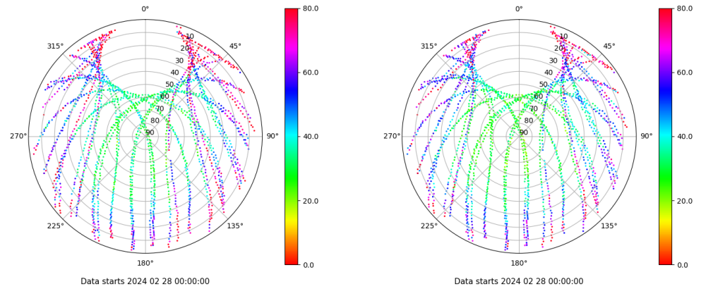
Skyplot for station BUIT. Parameter M1C Data file BUIT00ESP_R_2024059.xtr Skyplot for station BUIT. Parameter M2C Data file BUIT00ESP_R_2024059.xtr
