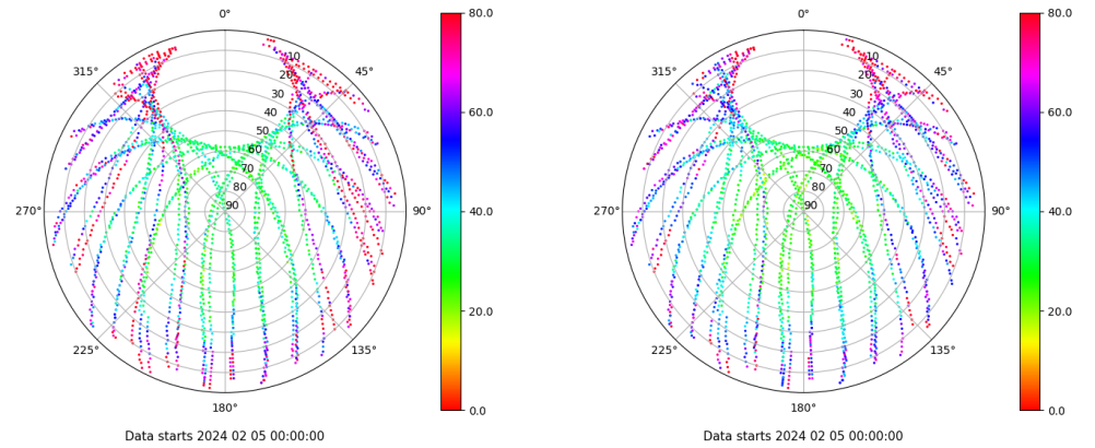
Skyplot for station BUIT. Parameter M1C Data file BUIT00ESP_R_2024036.xtr Skyplot for station BUIT. Parameter M2C Data file BUIT00ESP_R_2024036.xtr
