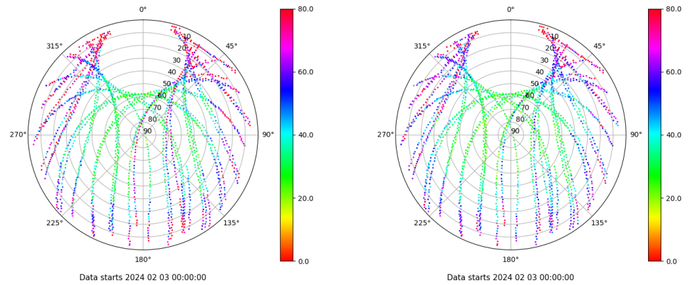
Skyplot for station BUIT. Parameter M1C Data file BUIT00ESP_R_2024034.xtr Skyplot for station BUIT. Parameter M2C Data file BUIT00ESP_R_2024034.xtr
