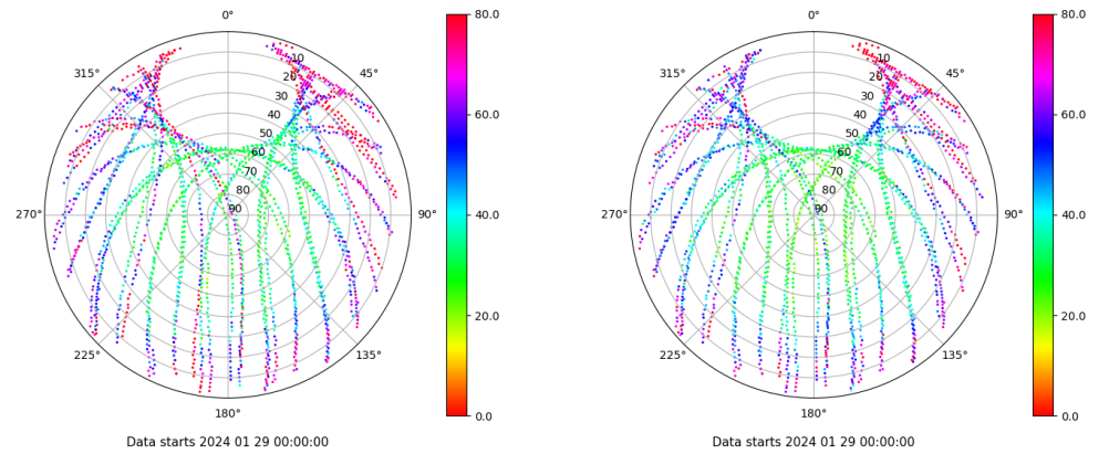
Skyplot for station BUIT. Parameter M1C Data file BUIT00ESP_R_2024029.xtr Skyplot for station BUIT. Parameter M2C Data file BUIT00ESP_R_2024029.xtr
