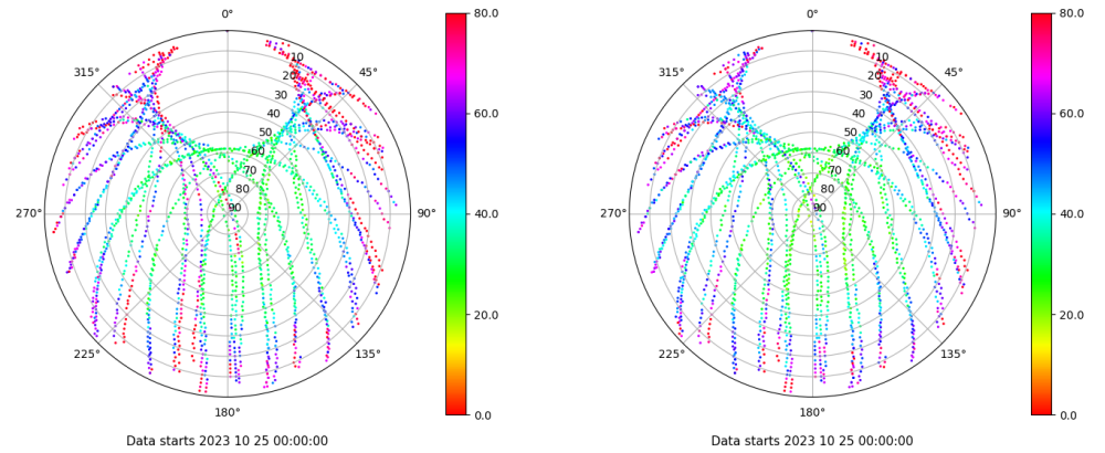
Skyplot for station BUIT. Parameter M1C Data file BUIT00ESP_R_2023298.xtr Skyplot for station BUIT. Parameter M2C Data file BUIT00ESP_R_2023298.xtr
