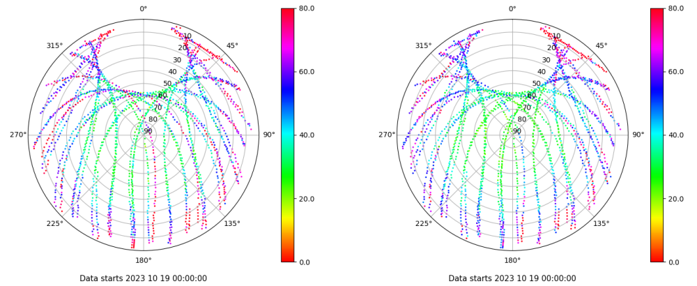
Skyplot for station BUIT. Parameter M1C Data file BUIT00ESP_R_2023292.xtr Skyplot for station BUIT. Parameter M2C Data file BUIT00ESP_R_2023292.xtr
