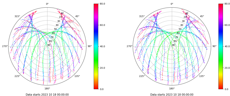
Skyplot for station BUIT. Parameter M1C Data file BUIT00ESP_R_2023291.xtr Skyplot for station BUIT. Parameter M2C Data file BUIT00ESP_R_2023291.xtr
