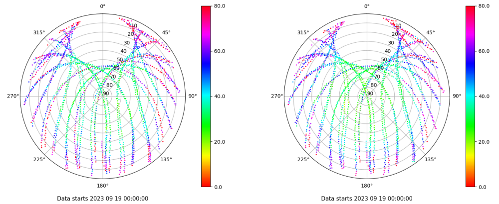
Skyplot for station BUIT. Parameter M1C Data file BUIT00ESP_R_2023262.xtr Skyplot for station BUIT. Parameter M2C Data file BUIT00ESP_R_2023262.xtr
