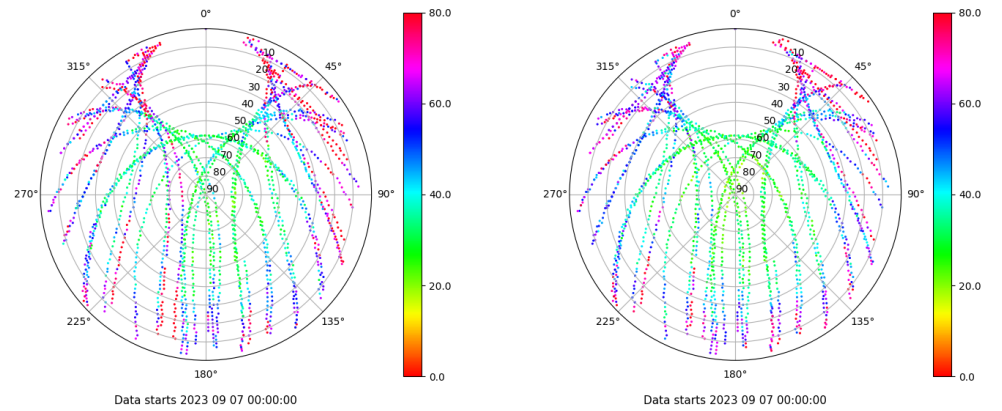
Skyplot for station BUIT. Parameter M1C Data file BUIT00ESP_R_2023250.xtr Skyplot for station BUIT. Parameter M2C Data file BUIT00ESP_R_2023250.xtr
