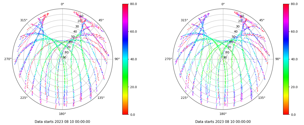
Skyplot for station BUIT. Parameter M1C Data file BUIT00ESP_R_2023222.xtr Skyplot for station BUIT. Parameter M2C Data file BUIT00ESP_R_2023222.xtr
