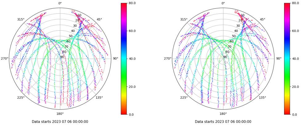
Skyplot for station BUIT. Parameter M1C Data file BUIT00ESP_R_2023187.xtr Skyplot for station BUIT. Parameter M2C Data file BUIT00ESP_R_2023187.xtr
