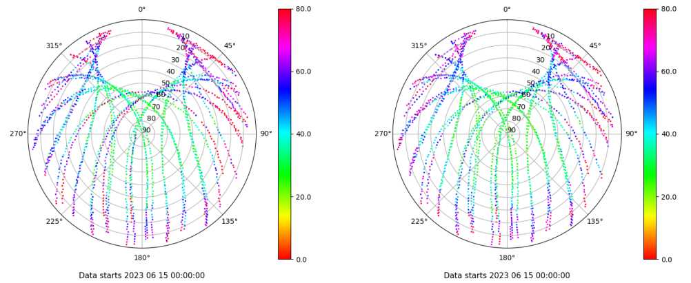
Skyplot for station BUIT. Parameter M1C Data file BUIT00ESP_R_2023166.xtr Skyplot for station BUIT. Parameter M2C Data file BUIT00ESP_R_2023166.xtr
