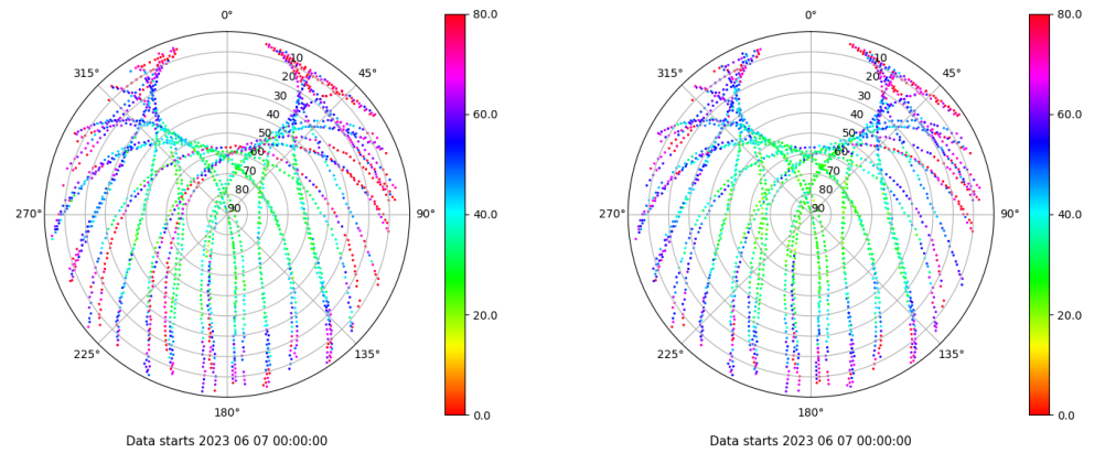
Skyplot for station BUIT. Parameter M1C Data file BUIT00ESP_R_2023158.xtr Skyplot for station BUIT. Parameter M2C Data file BUIT00ESP_R_2023158.xtr
