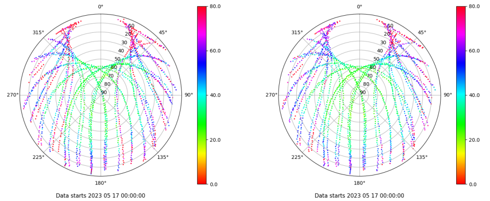
Skyplot for station BUIT. Parameter M1C Data file BUIT00ESP_R_2023137.xtr Skyplot for station BUIT. Parameter M2C Data file BUIT00ESP_R_2023137.xtr
