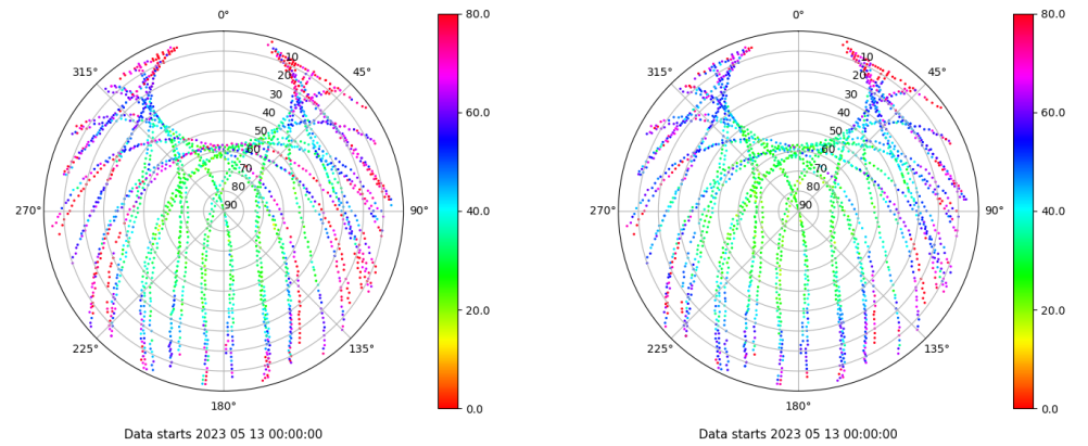
Skyplot for station BUIT. Parameter M1C Data file BUIT00ESP_R_2023133.xtr Skyplot for station BUIT. Parameter M2C Data file BUIT00ESP_R_2023133.xtr
