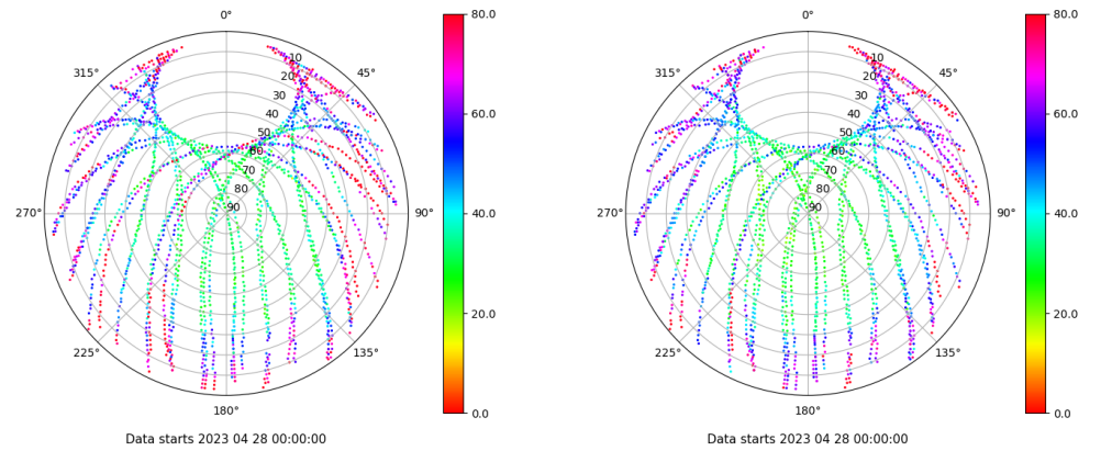
Skyplot for station BUIT. Parameter M1C Data file BUIT00ESP_R_2023118.xtr Skyplot for station BUIT. Parameter M2C Data file BUIT00ESP_R_2023118.xtr
