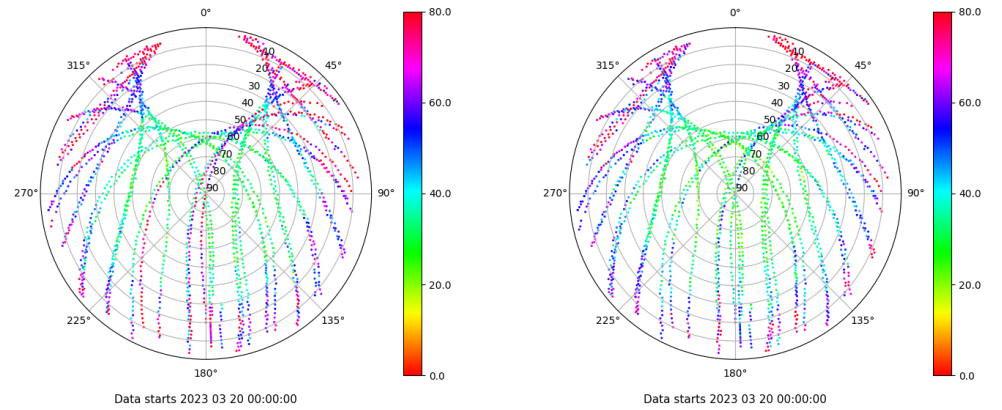
Skyplot for station BUIT. Parameter M1C Data file BUIT00ESP_R_2023079.xtr Skyplot for station BUIT. Parameter M2C Data file BUIT00ESP_R_2023079.xtr
