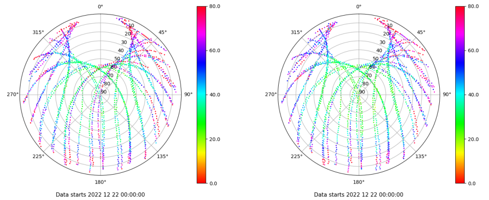
Skyplot for station BUIT. Parameter M1C Data file BUIT00ESP_R_2022356.xtr Skyplot for station BUIT. Parameter M2C Data file BUIT00ESP_R_2022356.xtr
