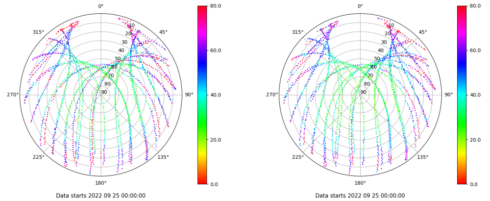
Skyplot for station BUIT. Parameter M1C Data file BUIT00ESP_R_2022268.xtr Skyplot for station BUIT. Parameter M2C Data file BUIT00ESP_R_2022268.xtr
