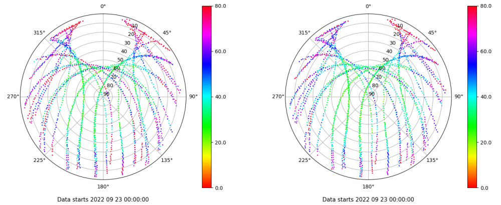
Skyplot for station BUIT. Parameter M1C Data file BUIT00ESP_R_2022266.xtr Skyplot for station BUIT. Parameter M2C Data file BUIT00ESP_R_2022266.xtr
