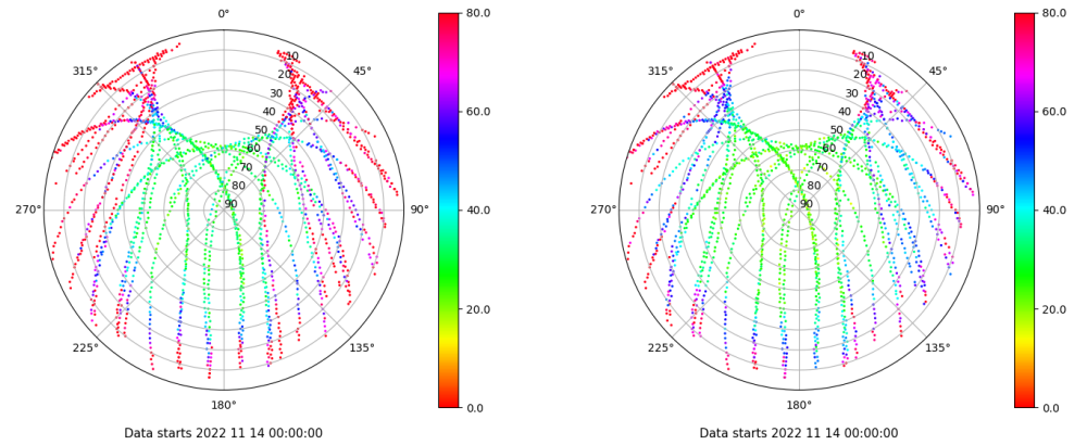
Skyplot for station BEJR. Parameter M1C Data file BEJR00ESP_R_2022318.xtr Skyplot for station BEJR. Parameter M2C Data file BEJR00ESP_R_2022318.xtr
