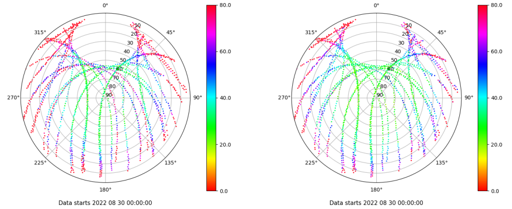
Skyplot for station BEJR. Parameter M1C Data file BEJR00ESP_R_2022242.xtr Skyplot for station BEJR. Parameter M2C Data file BEJR00ESP_R_2022242.xtr
