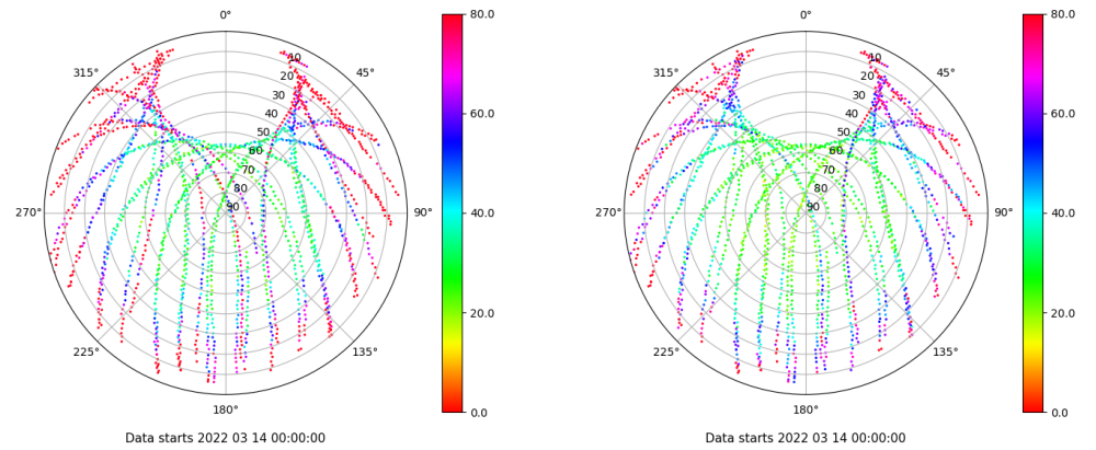
Skyplot for station BEJR. Parameter M1C Data file BEJR00ESP_R_2022073.xtr Skyplot for station BEJR. Parameter M2C Data file BEJR00ESP_R_2022073.xtr
