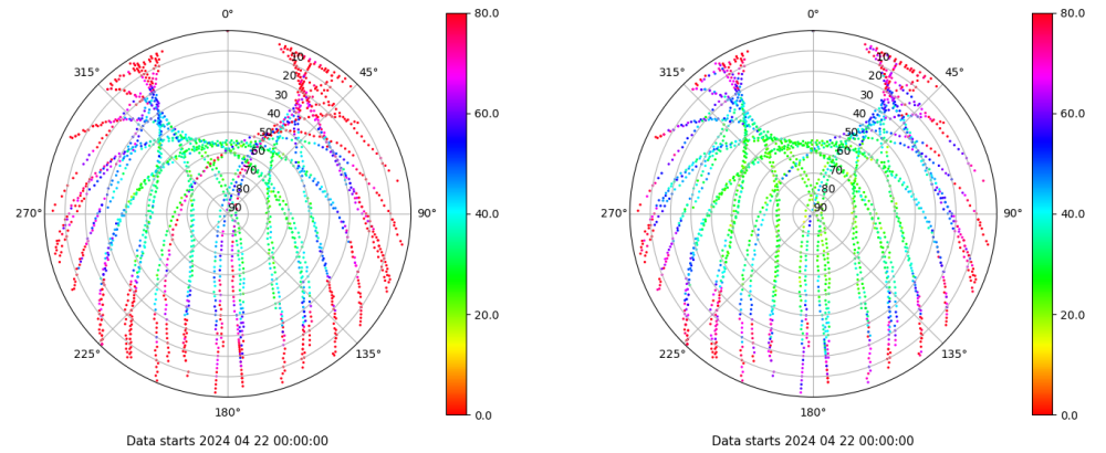
Skyplot for station BADI. Parameter M1C Data file BADI00ESP_R_2024113.xtr Skyplot for station BADI. Parameter M2C Data file BADI00ESP_R_2024113.xtr
