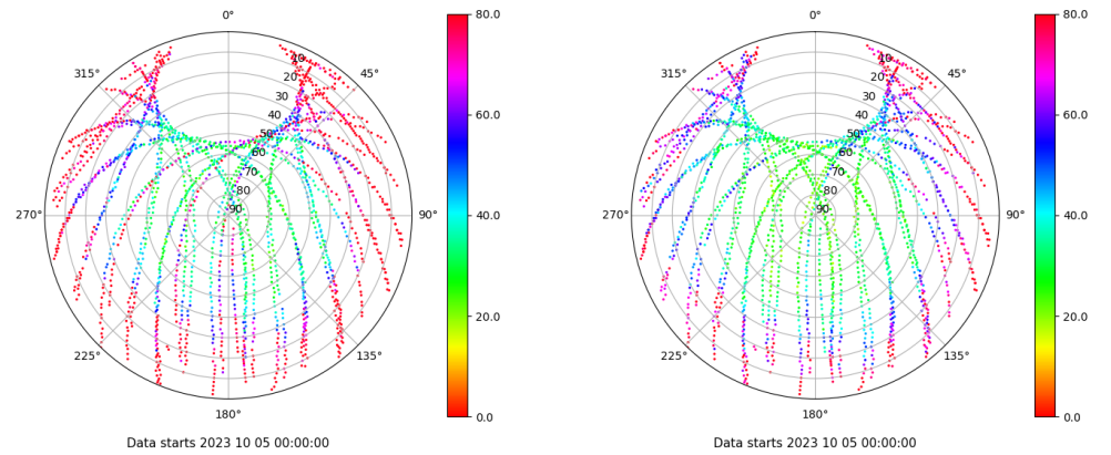
Skyplot for station BADI. Parameter M1C Data file BADI00ESP_R_2023278.xtr Skyplot for station BADI. Parameter M2C Data file BADI00ESP_R_2023278.xtr
