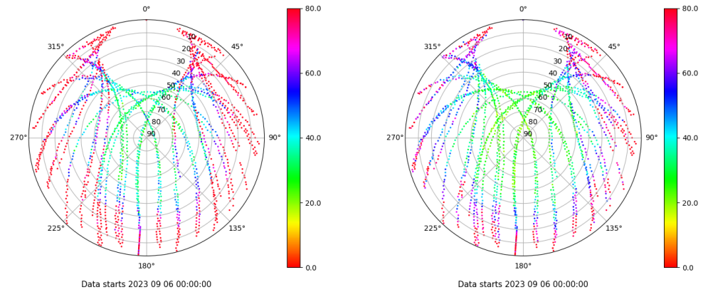
Skyplot for station BADI. Parameter M1C Data file BADI00ESP_R_2023249.xtr Skyplot for station BADI. Parameter M2C Data file BADI00ESP_R_2023249.xtr
