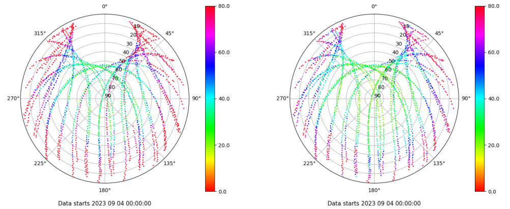
Skyplot for station BADI. Parameter M1C Data file BADI00ESP_R_2023247.xtr Skyplot for station BADI. Parameter M2C Data file BADI00ESP_R_2023247.xtr
