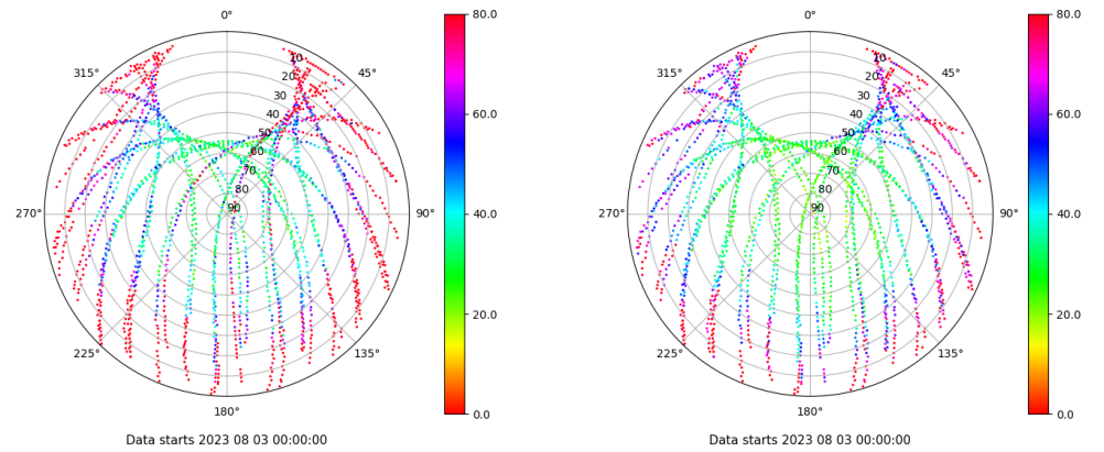
Skyplot for station BADI. Parameter M1C Data file BADI00ESP_R_2023215.xtr Skyplot for station BADI. Parameter M2C Data file BADI00ESP_R_2023215.xtr
