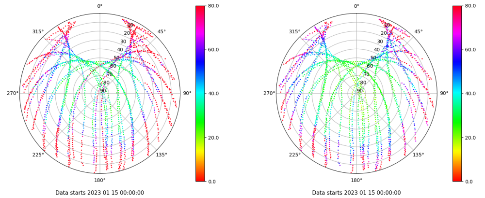
Skyplot for station BADI. Parameter M1C Data file BADI00ESP_R_2023015.xtr Skyplot for station BADI. Parameter M2C Data file BADI00ESP_R_2023015.xtr
