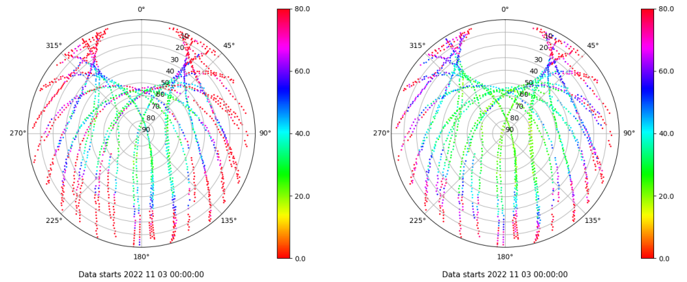
Skyplot for station BADI. Parameter M1C Data file BADI00ESP_R_2022307.xtr Skyplot for station BADI. Parameter M2C Data file BADI00ESP_R_2022307.xtr
