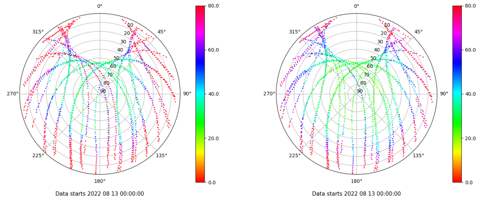
Skyplot for station BADI. Parameter M1C Data file BADI00ESP_R_2022225.xtr Skyplot for station BADI. Parameter M2C Data file BADI00ESP_R_2022225.xtr
