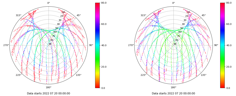
Skyplot for station BADI. Parameter M1C Data file BADI00ESP_R_2022201.xtr Skyplot for station BADI. Parameter M2C Data file BADI00ESP_R_2022201.xtr
